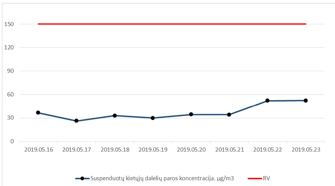
2 pav. Vidutinē paros SKD koncentrācija KLASCO teritorijojē N. Uosto g. 23
